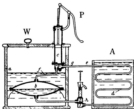
W：コンデンサー，A：エバポレーター（A中の水を氷にすることができる），h：膨張弁 図 パーキンスのエーテル機（参考文献 [2]，p. 20）
