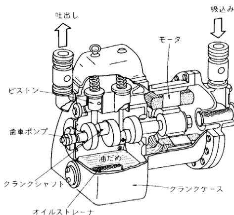
図 往復式圧縮機の例（参考文献 [5], p.126）
