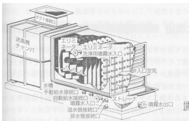
図 エアワッシャーの例（参考文献 [3], p. 75）
