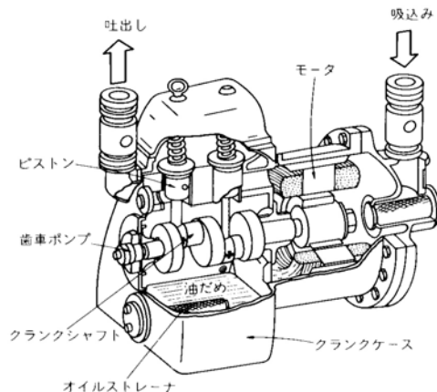
図 往復式圧縮機の例（参考文献 [4], p. 126）
