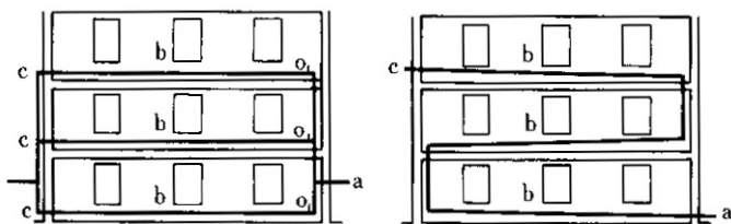
a：蒸気管 b：放熱管
