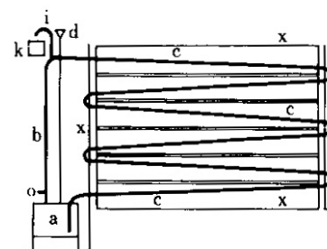
a：ボイラ d：開放式膨張タンク
