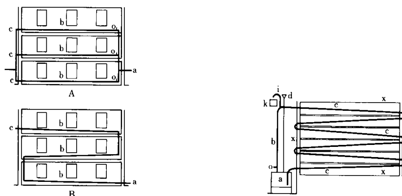
図 鋳鉄管を用いた一管式蒸気暖房（参考文献3）
