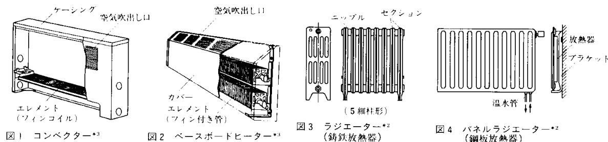
図 放熱器のいろいろ（参考文献5）
