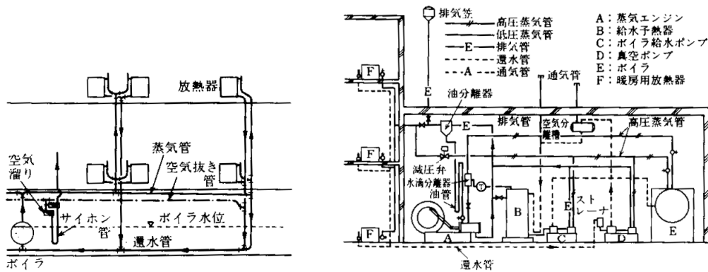
図 ケルチング式蒸気暖房（参考文献3） 図 ウェブスター式蒸気暖房（参考文献3）
