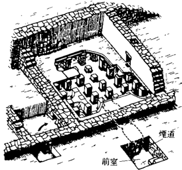
図 ローマ時代のハイポコースト暖房概略図（参考文献2）
