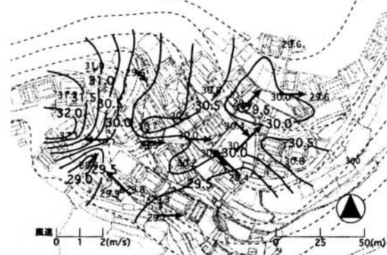
図7 27日 16:00の気温と風向・風速の分布
