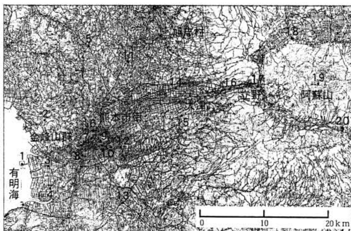
図1 熊本地域と各観測地点の位置
