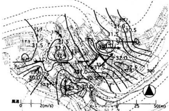
図11 29日 16:00の気温と風向・風速の分布
